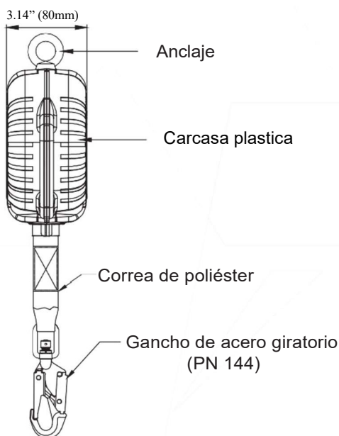
VISTA LATERAL
